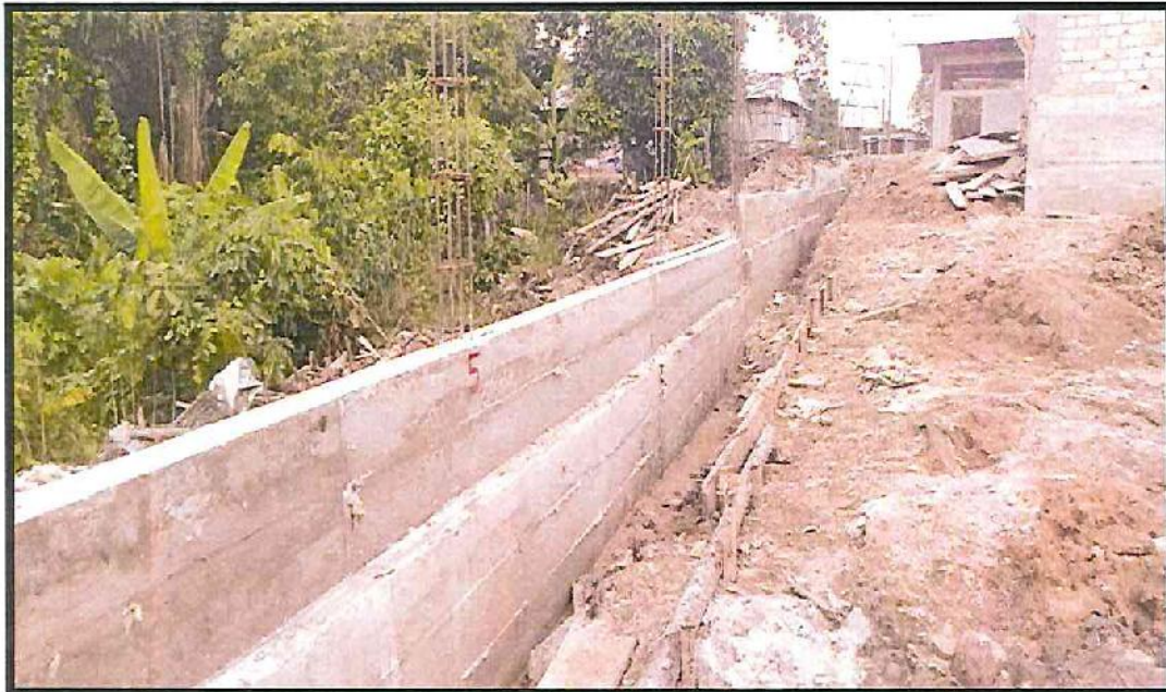
CIMIENTO Y SOBRECIMIENTO
