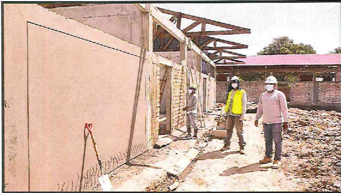
TARRAJEO EXTERIOR EN MODULO 1
