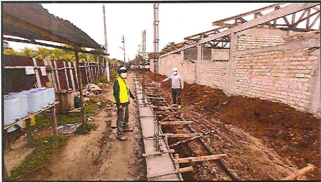
PLANTADO DE COLUMNAS Y VACEO EN CIMENTO CORRIDO
