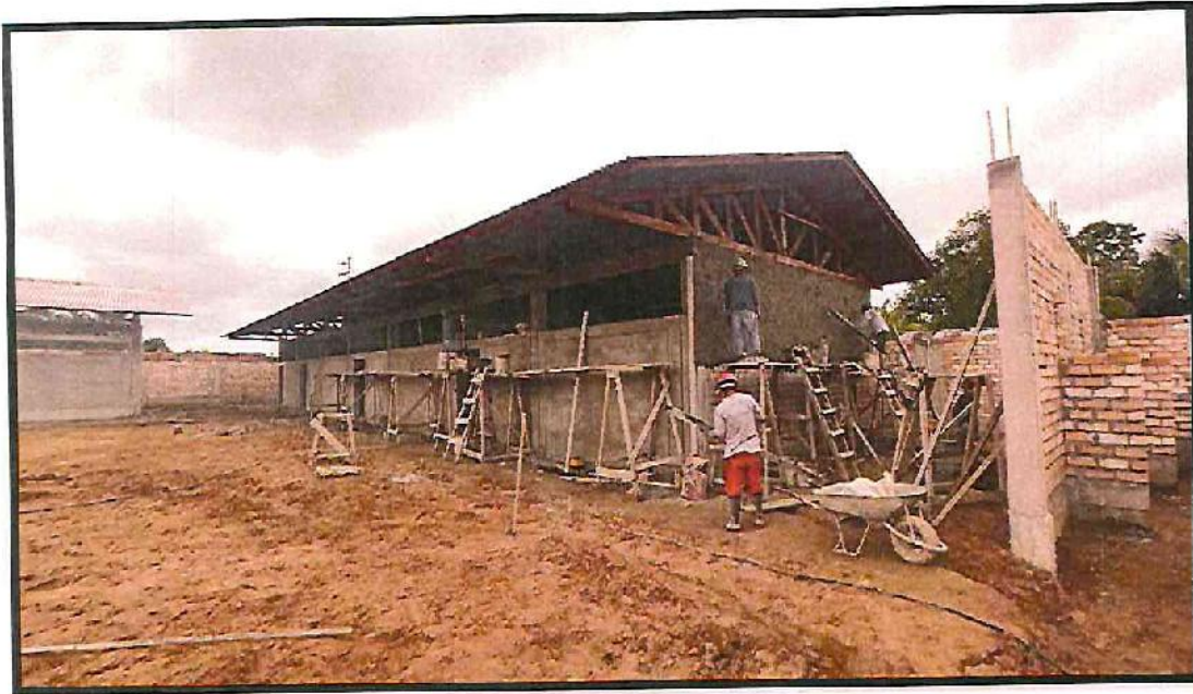
TARRAJEO EXTERIOR Y DERRAMES EN MODULO 2
