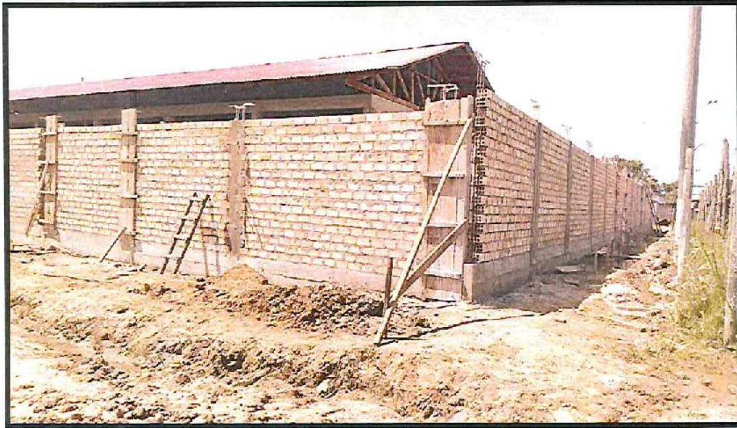
MURO DE LADRILLO TIPO SOGA
